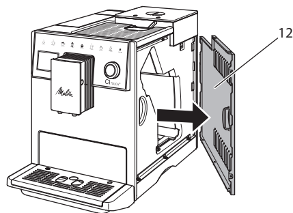
Joon. 13: Külgmise kate mahavõtmine
